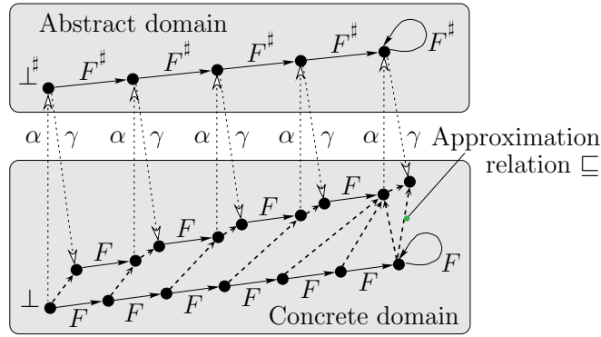
Fig. 10. Fixpoint Abstraction \text{lfp } F \sqsubseteq \gamma(\text{lfp } F^\#)
